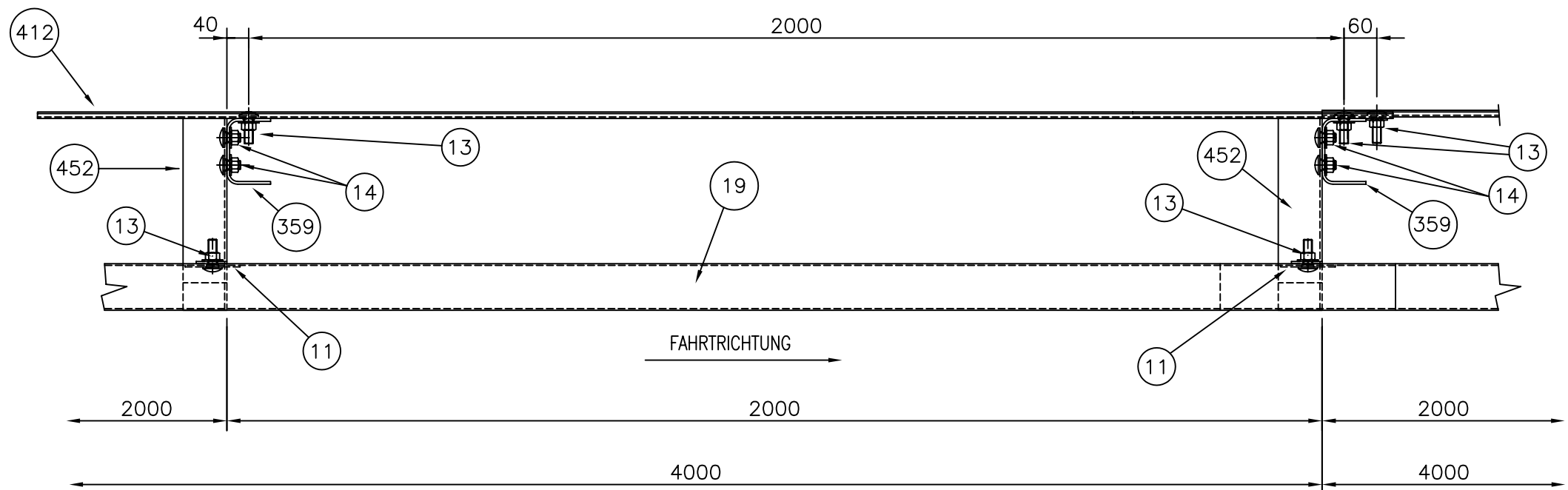
ANSICHT A-A
